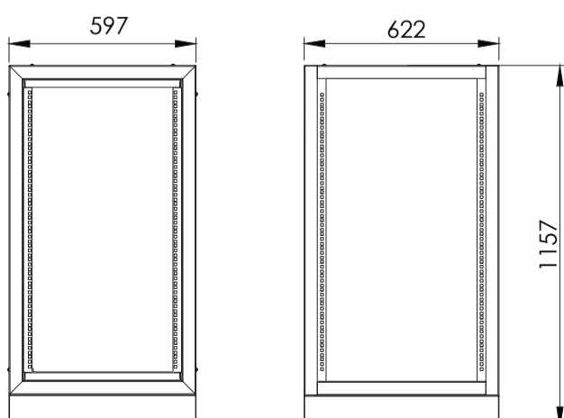
Dimensiones generales
